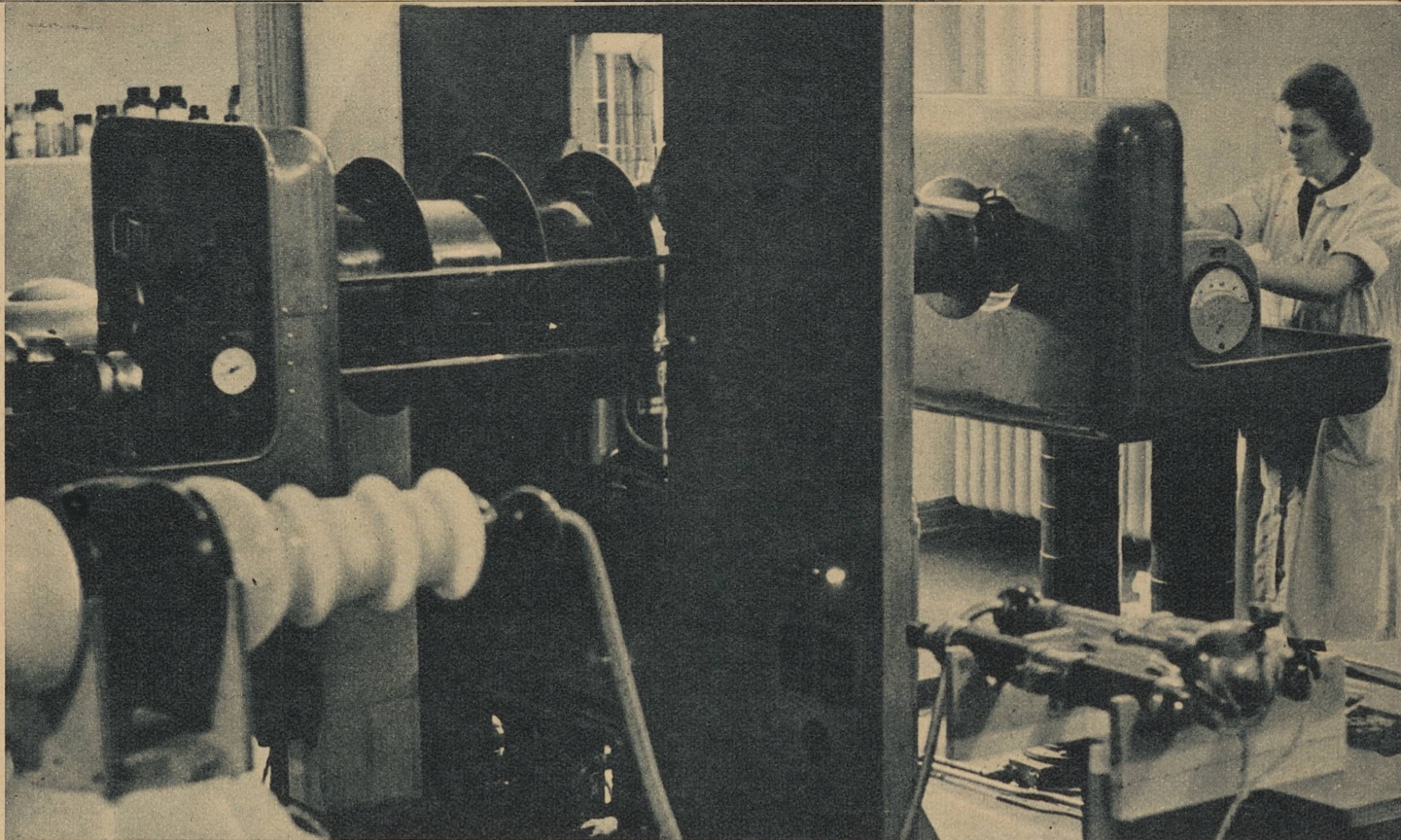
HER SKYTES MED SKARPT. Det med 600 000 volt arbeidende høyspenningsanlegg i Keiser-Wilhelm-instituttet for kjemi produserer nevtronstråler. Disse konsentreres på det medikament, hvis virkeverne man vil undersøke — i dette tilfelle kalk — og deres energi gjør det radioaktivt, d.v.s. selvstrålende
