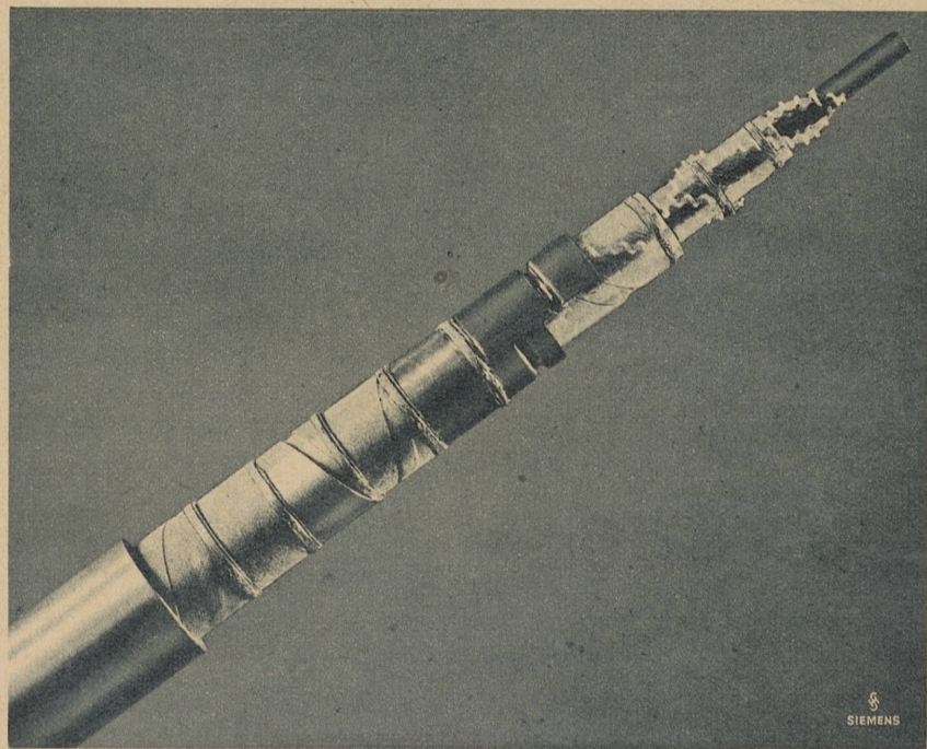
Bredbåndkabel i Siemens & Halskes byggeutførelse (Werkbild Siemens)
