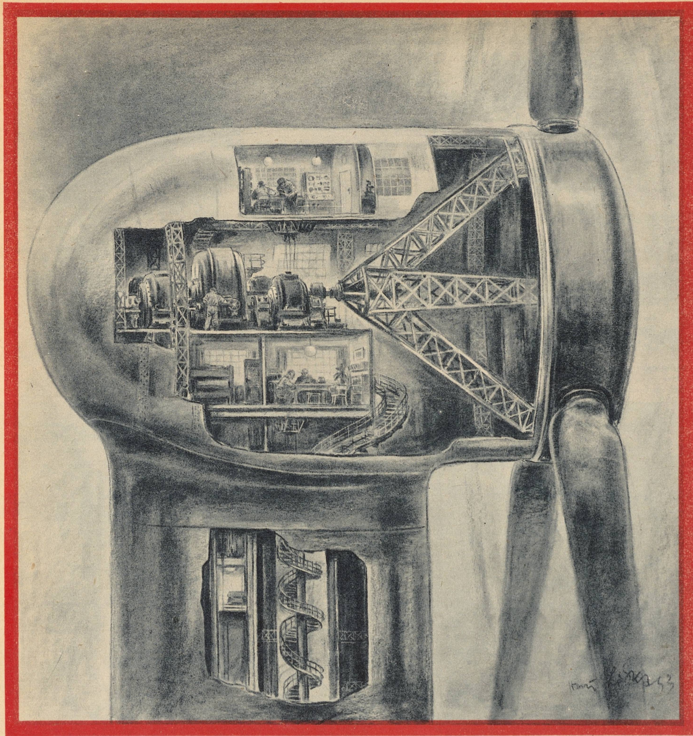
En kraftstasjon — 250 meter over jorden! Bildet viser et tverrsnitt gjennom et av de kjempemessige vindkraftverk som artikkelen her handler om. På toppen av kraftverkets kjempetårn — som av og til er utsatt for en vind, der på jorden vilde få kraftige trær til å svaie — er det anbrakt en gondol med et veldig vingehjul. Gondolen er kjernen i anlegget, hvor vindens vilde kraft blir omvandlet til elektrisitet. Den er 45 meter lang og 20 meter høy. De tre etasjer omfatter maskinrom, et meteorologisk observatorium og oppholdsrom for kraftverk-personalet. Det trengs ikke mer enn 5—8 mann til betjening. Det trevingede svinghjul har en diameter av 135 meter. Det gjør 10 omdreininger i minuttet; vingespissene har da en omdreiningshastighet av 260 kilometer i timen. I gondolens indre blir hjulets omdreininger omsatt i hurtighet og overført på fire dynamo-maskiner. Den produserte elektriske energi blir gjennom tykke kabler gjennom tårnets indre ledet ned i en transformator som er tilsluttet strømmettet. En person- og en vareheis samt en vindeltrapp forbinde kraftstasjonen oppe i luften med jorden
